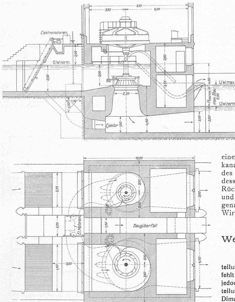
Abb. 8 bis 10. Moderne Konursturbinen-Anlage. — Schnitte 1:20.
