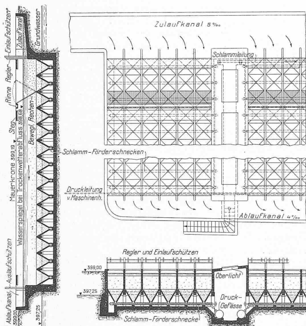
Abb. 3. Grundriss und Schnitte der Klärinnen. — 1 : 250.
