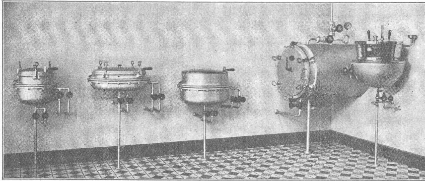
Komplette Sterilisieranlage, bestehend aus Instrumenten- und Tuppersterilisator, Waschbeckenkocher, Verbandstoff- und Wassersterilisierapparaten
