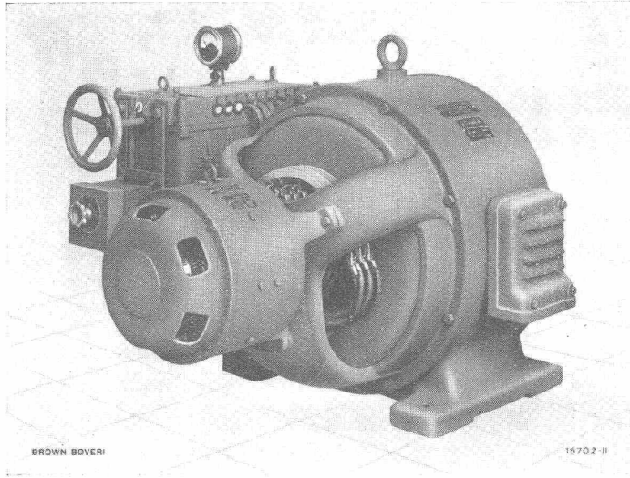
Dreiphasen-Synchron-Induktions-Mo'tor, 118 kW, Drehzahl 1000, \cos \varphi = 0,98 voreilend.
