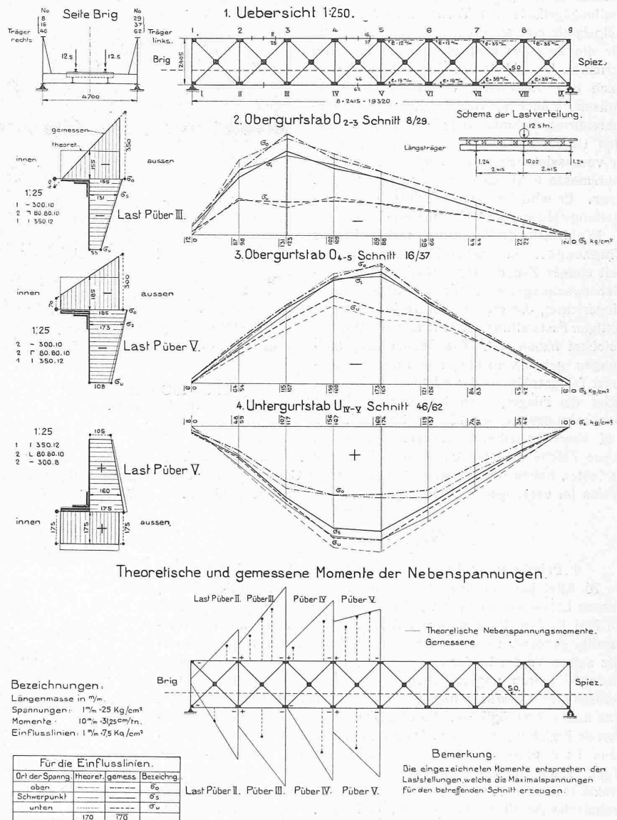
Abb. 22. Suldbachbrücke bei Mülten-Aeschi, Kt. Bern. — Bern-Lötschberg-Simplon-Bahn.
