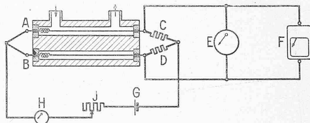
Abb. 1. Schema des elektrischen Rauchgasprüfers, System Siemens & Halske, nebst zugehörigen Instrumenten.
