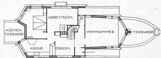
Abb. 29 und 30. Grundrisse und Aufriss zu Abb. 23. — Etwa 1 : 300.
