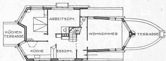
Abb. 29 und 30. Grundrisse und Aufriss zu Abb. 23. — Etwa 1 : 300.
