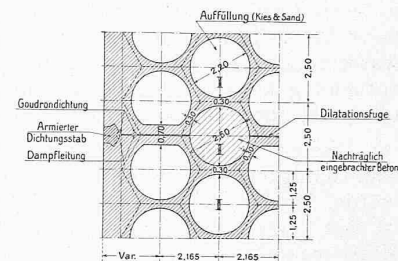
Abb. 5. Fugendichtung 1:250.
