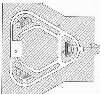
Coupees horizontale et verticale du four électrique à induction.
