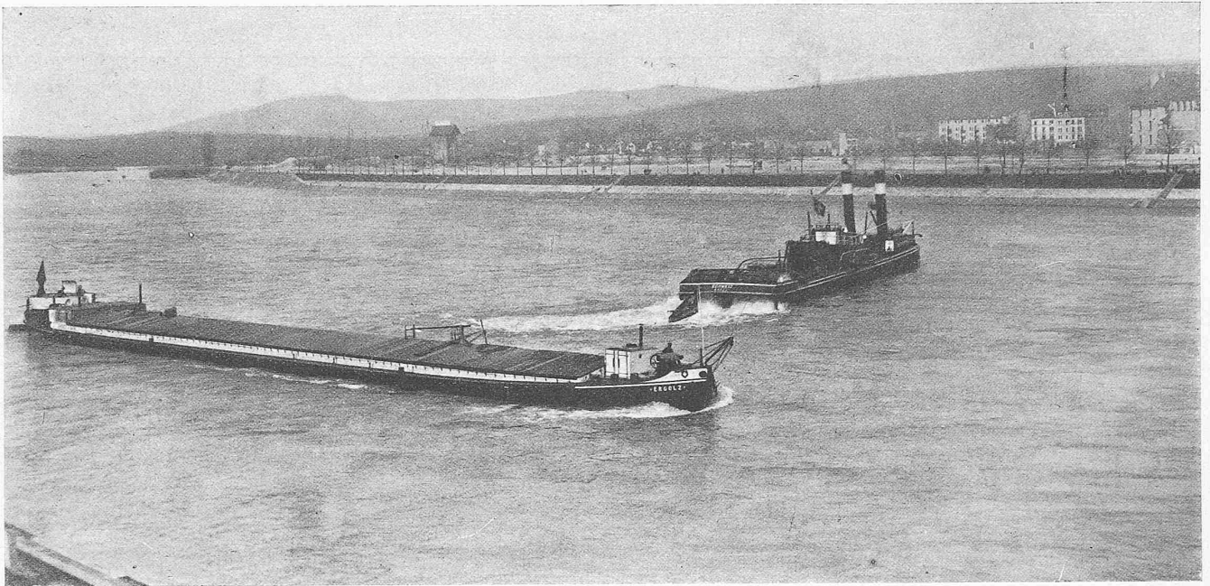
Abb. 1. Wendung zur Talfahrt des Heckraddampfers „Schweiz“ (750 PS, erbaut 1919) mit dem Kahn „Ergolz“ der Schweizer Schlepsschiffahrts-Genossenschaft.
