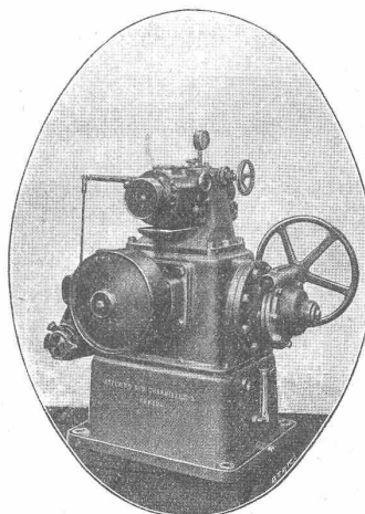
RÉGULATEUR DE VITESSE BREVETÉ MODÈLE 1923
