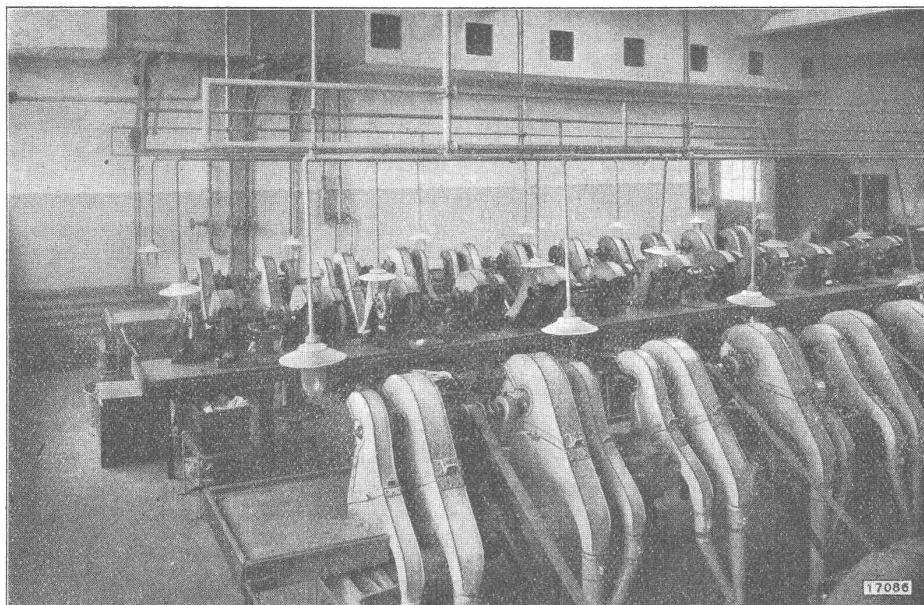
Entstaubung in einer Zelluloidwarenfabrik. Mit Hilfe von Spezialvorrichtungen wird die Gefahr einer Explosion des Zelluloidstaubes vollständig beseitigt.
