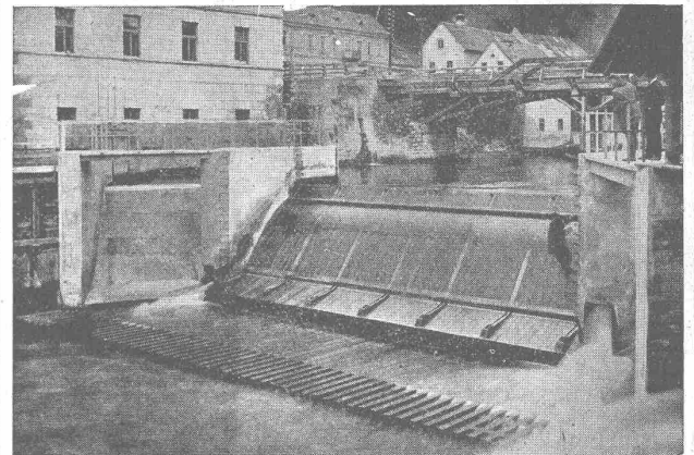
Dachwehre in der Mürz der Kabelwerke Felten & Guillaume, Bruck a. d. Mur.
