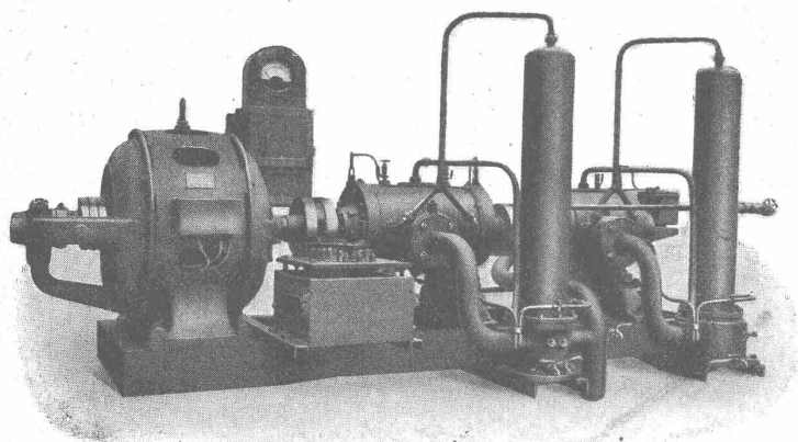
Leicht transportable Kompressoranlage für 5–10 Atm. Druck
