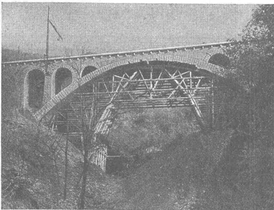
SBB Monte Ceneri, Selvacciabücke, 42,20 m weit.
