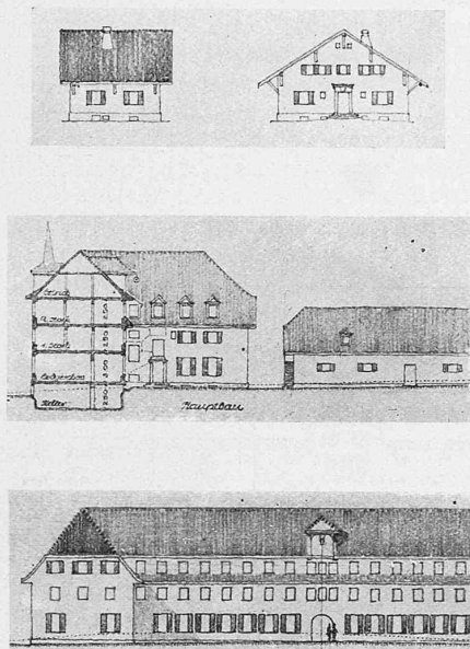
Oben Direktionshaus; darunter Schnitt und Hoffront des Hauptgebäudes 1:800. — Fliegerbild aus Südost.
