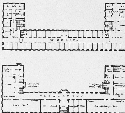
Entwurf Nr. 1. Grundrisse vom Hauptbau 1:800. Lageplan 1:3000, mit 1 m-Kurven.
