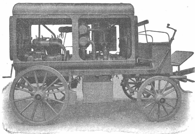
Fahrbare Kompressor-Anlage
