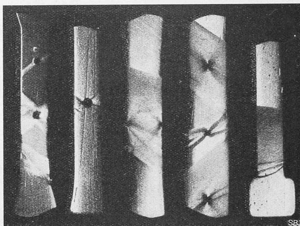
Abb. 36 bis 40. Fliessfiguren auf gelochten und gekerbten Zugstäben aus Eisen. Lokale, scharfe Gleitlinienbildung, matte breite Fließstreifen.
