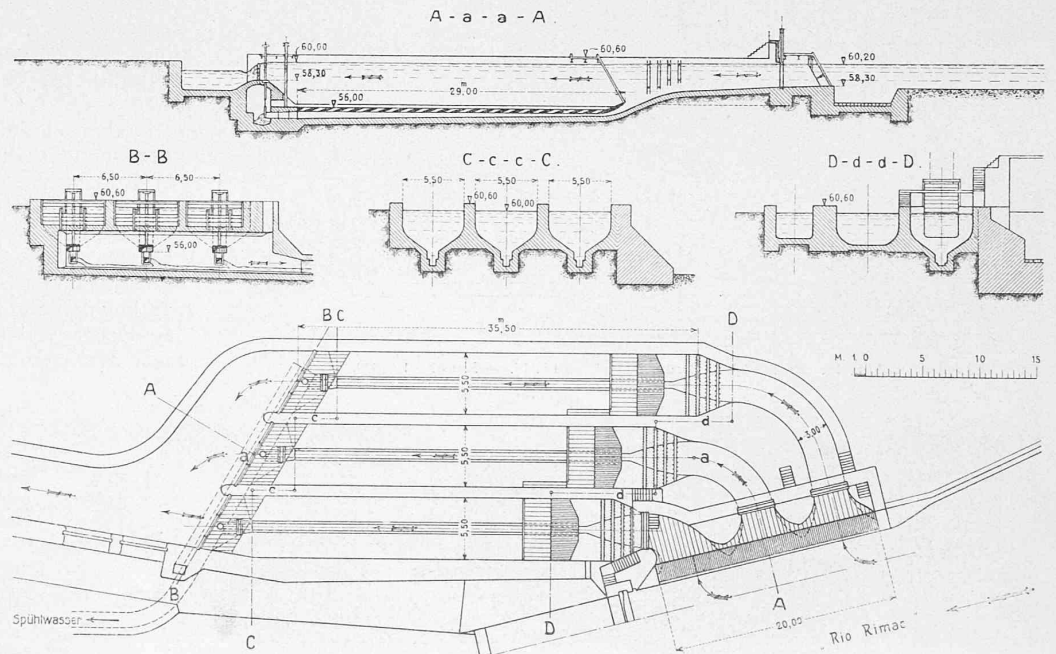
Abb. 7. Automatischer Entsander des Kraftwerkes Yanacoto am Rio Rimac, 15 000 PS Q = 20 m 3 /sek, H = 72 bis 75 m. - 1:600.
