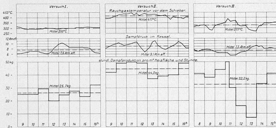
Abb. 17. Graphische Darstellung des Verlaufs der an obiger Anlage vorgenommenen Verdampfungsversuche.
