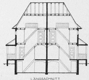
Abb. 5. Schnitt zu Abb. 4 (unten).
