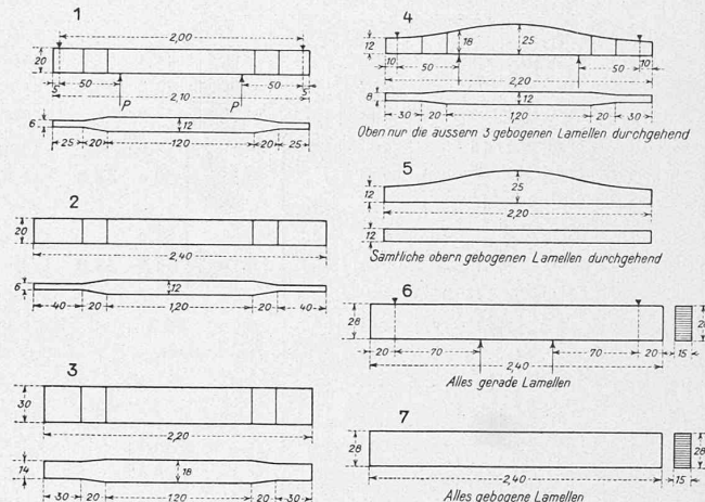
Abb. 1. Typen der untersuchten Balken.
