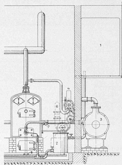
Abb. 32. Anordnung einer Heizanlage mit Oelfeuerung Bauart Cuénod.
