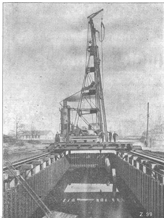
Rötibrücke Solothurn (Ausführung in Gemeinschaftsunternehmung) Fundierung des Flusspfeilers
