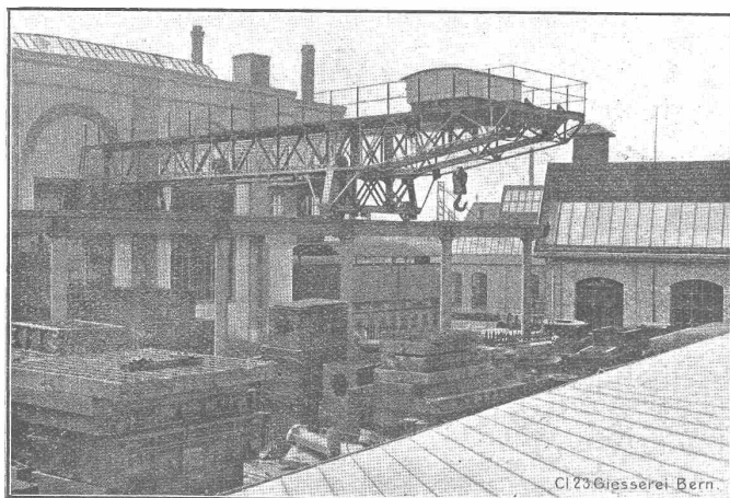
Hof-Lauikran, Tragkraft 15 Tonnen, Länge 23 m, mit einseitigem festen Ausleger.
