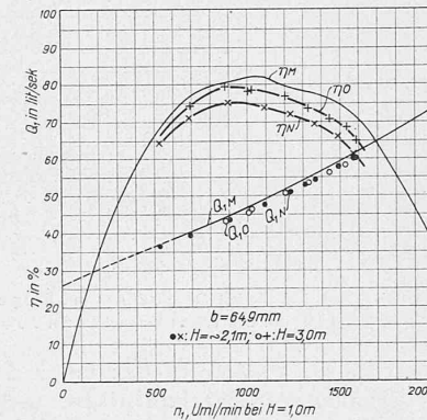
Abb. 31. Versuche mit Modell D_s = 167 mm.
