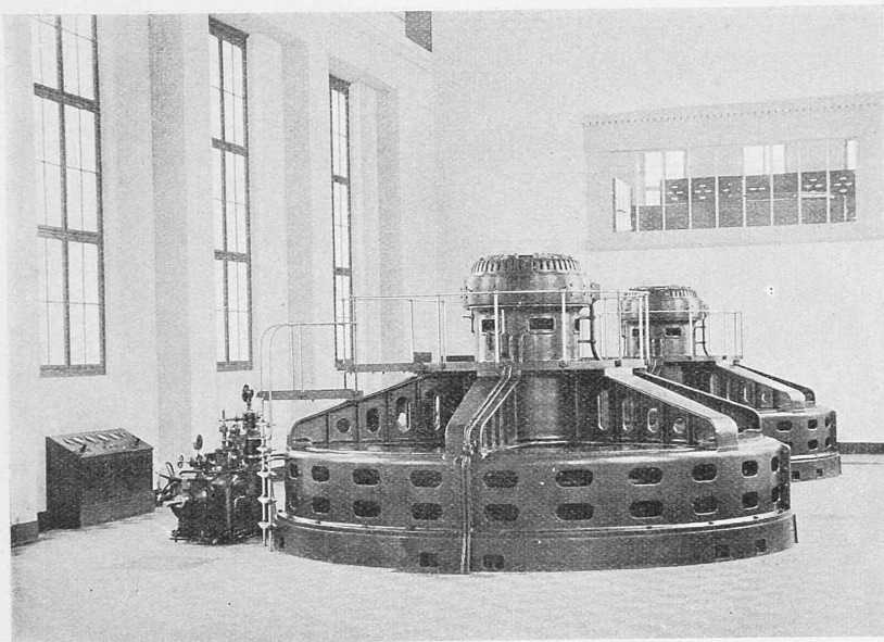
Abb. 6. Innenansicht des Maschinensaales mit den 2200 kVA-Generatoren von Brown, Boveri &amp; Cie.
