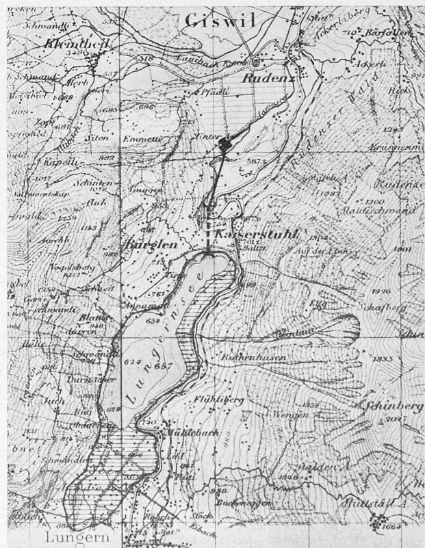
Abb. 1. Uebersichtsplan des Lungernsee-Kraftwerks. — Masstab 1:50 000 Mit Bewilligung der Schweizer. Landestopographie vom 30. Sept. 1921.
