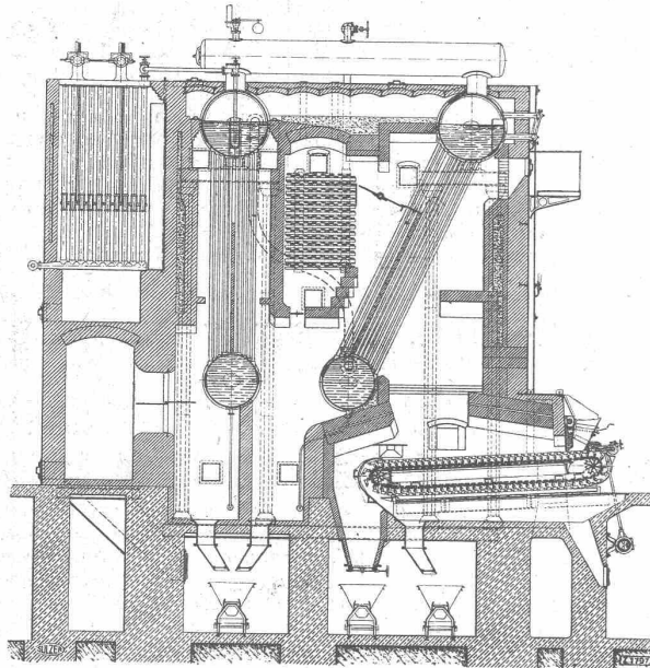
Sulzer-Steilrohrkessel (Patentiert)
