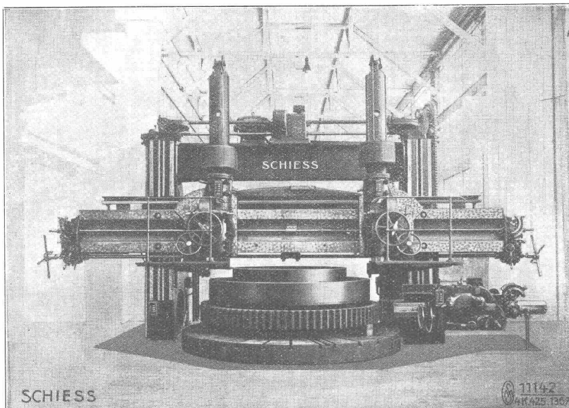
Schwere Karusselldrehbank mit 4250 mm Drehdurchmesser. Diese Maschine besitzt Balligdrehvorrichtung und ist mit elektrischer Druckknopfsteuerung ausgerüstet.
