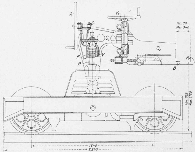
Abb. 1. Skizze des „Locomoteur Vermot“. Nach „Engineering“ vom 23. Dez. 1923.
