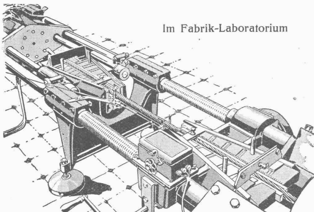
Drahtseil-Zerreiss-Versuch
