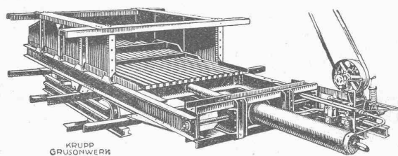
Schubrostentleerung für Kalk-Schachtföfen
