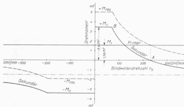
Abb. 12. Drehmomente an der Blindwelle des Zahnradgetriebes.
