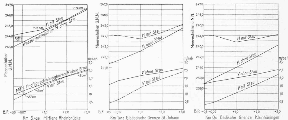
Abb. 9. Wasserspiegelhöhen H und Wassergeschwindigkeiten V in Funktion des Wasserstandes für drei Stellen der baselstädtischen Staustrecke (links Mittlere Rheinbrücke) mit und ohne Stau.
