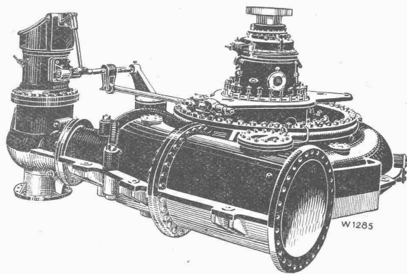
Wasserturbine für das Kraftwerk Wäggital
