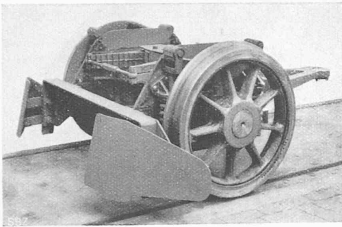
Abb. 7. Einachsiges Bisselgestell.
