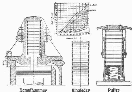
Dampfhammer
