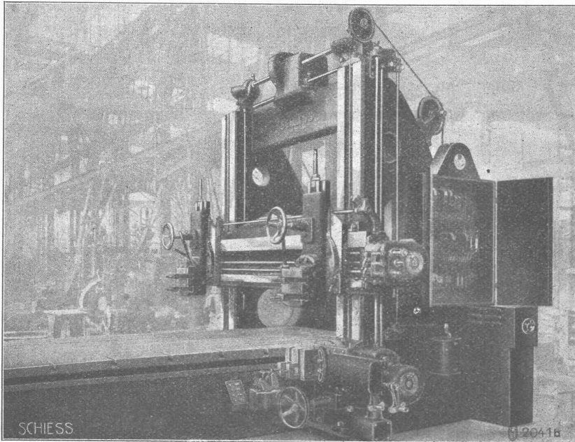
Tischhobelmaschinen
