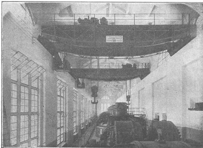
Zwei elektrische Laufrane von je 50 Tonnen Tragkraft in der Zentrale Mühleberg der Bernischen Kraftwerke A.-G.
