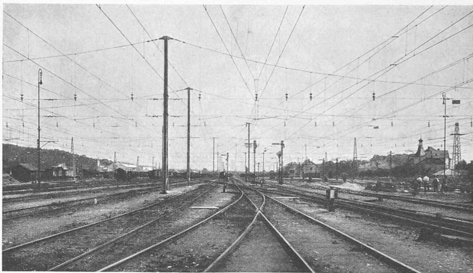
Abb. 7. Fahrdrabt-Aufhängung im Bahnhof Attnang-Puchheim. — A.E.G. Union E.G.
