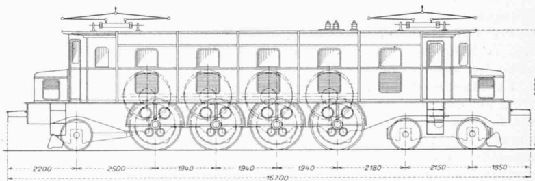
Abb. 21. Ae 1/2 Schnellzug-Lokomotive der S. B. B. für die Linie Lausanne-Vallorbe. — 1:150. Zurzeit im Bau bei Brown, Boveri & Cie. in Baden und der Lokomotivfabrik Winterthur.
