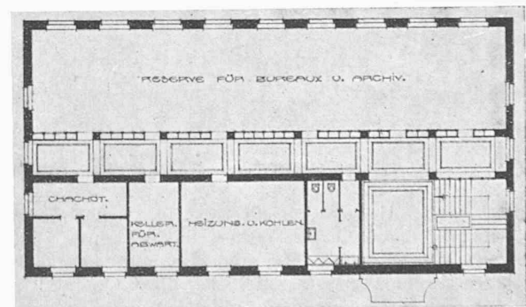
Untergeschoss, Erd- und Dachgeschoss, 1:350, zu Entwurf Nr. 9.
