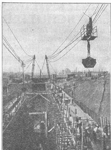
Bleichert-Kabelkrane beim Schleusenbau
