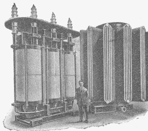
Drehstrom-Öltransformator von 13000 kVA, mit Ölkühlung 70000/13500 Volt
