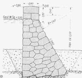
Abb. 2. Normalprofil der Staumauern. Masstab 1:100.
