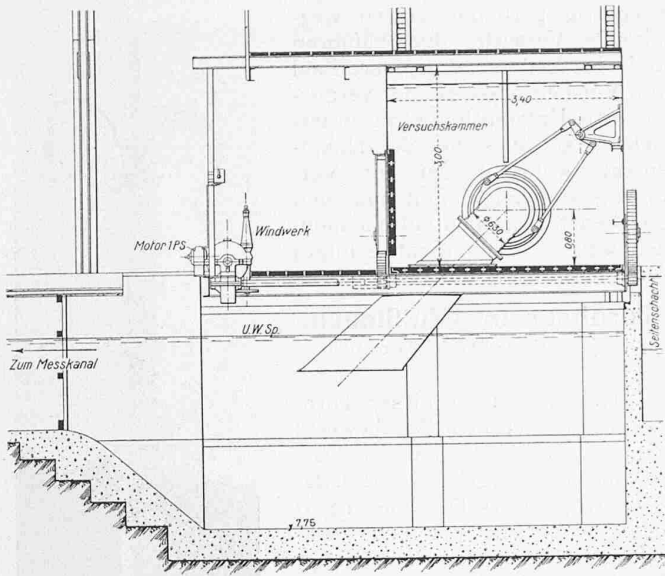
Abb. 26. Wandertrog in tiefster Lage, Francisturbine mit fliegendem Laufrad und schiefem Saugrohr, Turbinenaxe quer zur Kanalaxe — 1:100.
