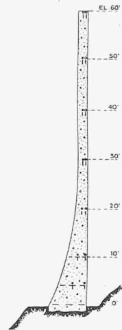
Abb. 3. Verteilung der horizontal, vertikal und radial einbetonierten elektrischen Spannungs- und Temperaturmesser (Wasserseitige Ansicht und Schnitt).
