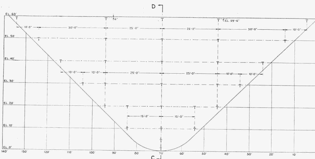
Abb. 3. Verteilung der horizontal, vertikal und radial einbetonierten elektrischen Spannungs- und Temperaturmesser (Wasserseitige Ansicht und Schnitt).
