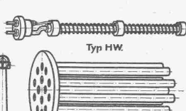
Einzelne elektrische Heizeinsätze zum Einbauen.
