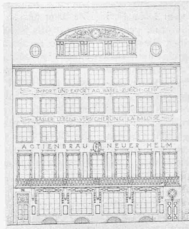
Abgeänderte Fassade.
