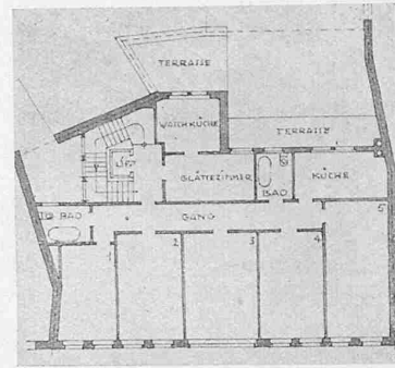
IV. Rang, Entwurf Nr. 2. — Verfasser Bercher & Tamm, Architekten, Basel. — Grundrisse vom Erdgeschoss sowie I. und IV. Obergeschoss. — 1:400.
