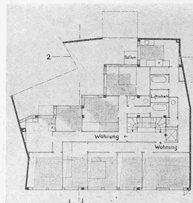
V. Rang, Entwurf Nr. 6. — Verfasser Hans Wittwer, Architekt, Basel. — Grundrisse vom Erdgeschoss, sowie I. und IV. Obergeschoss. — 1 : 400.
