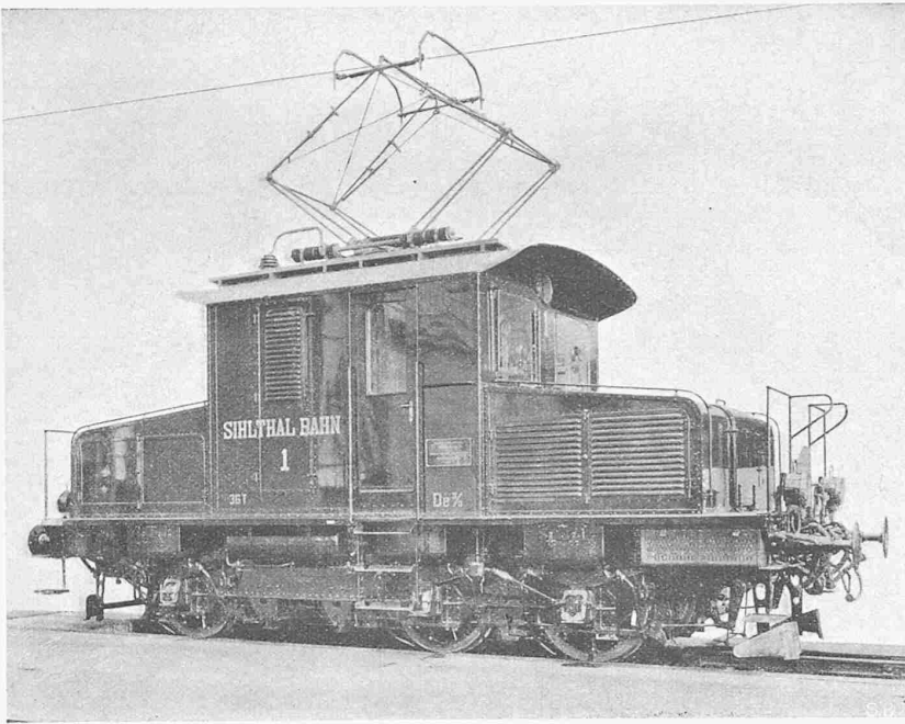
Abb. 1. D e 3/3-Güterzug-Lokomotive für 15000 V Einphasenwechselstrom der normalspurigen Sihlthalbahn.
