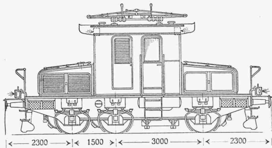
Abb. 1. Typenskizze der Sihlthalbahn-Lokomotive. — Masstab 1: 120.
