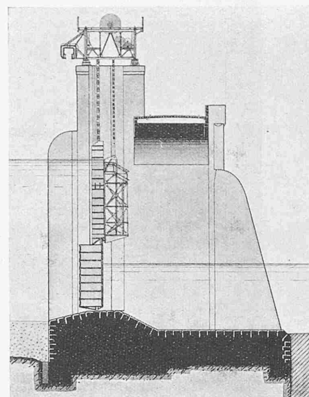
Abb. 14. Laufenburg 1908. Doppelschützen. — 1:500.
