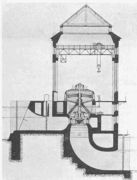
Abb. 18. Kraftwerk Eglisau, erbaut 1915/20. — Masstab 1 : 500. H max = 10,8 m; Q = 56,4 m 3 /sek, N = 6000 PS pro Turbine.
