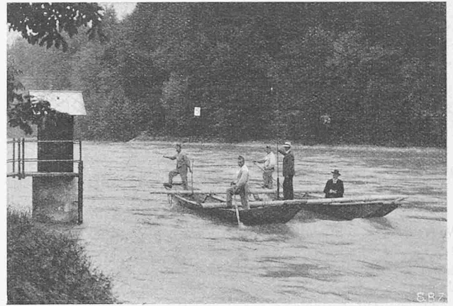
Abb. 6. Flügelmessung mit Stangenführung. (Aare bei Bern).
