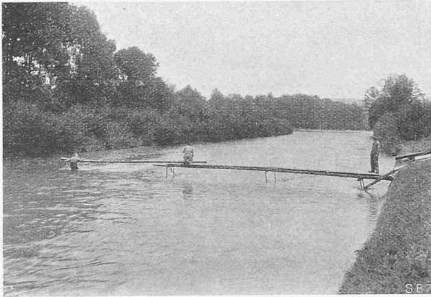
Abb. 5. Stegbau für eine Flügelmessung (Sitter bei Bischofszell).
