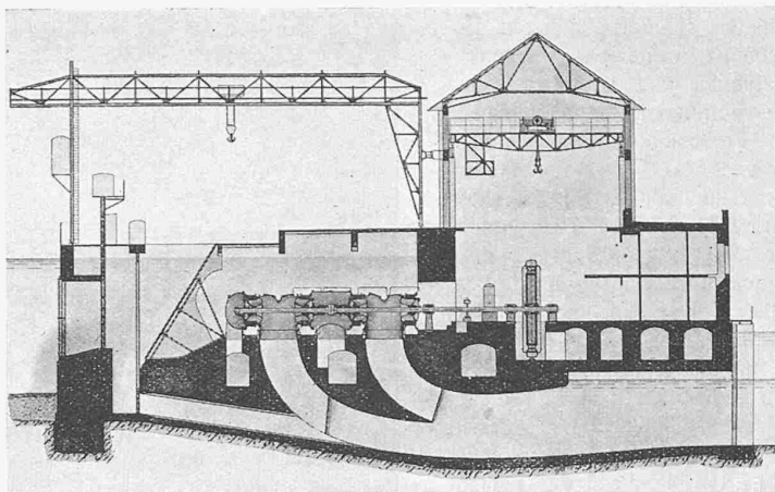
Abb. 17. Baselstädtisches Kraftwerk Augst, erbaut 1907/12. — Masstab 1 : 500. H max = 7,75 m; Q = 38 m 3 /sek, N = 3000 PS pro Turbine.
