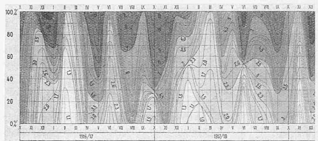
Abb. 4. Abfluss des Lauerzersees, 450 m ü. M., 1916/17 bis 1919/20. Einzugsgebiet: 72,1 km 2 . Mittlere Höhe: 887 m ü. M. Keine Vergletscherung.
