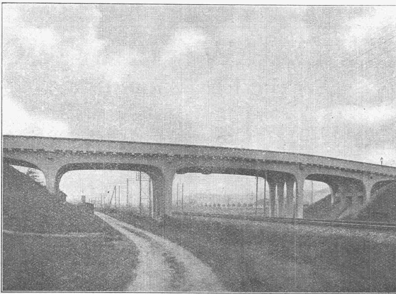
Strassenüberführung beim Gaswerk Schlieren (54 m lang)
