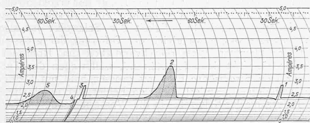
Abb. 2. Registrierstreifen.
