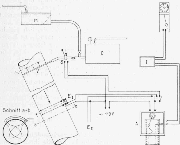
Abb. 1. Messanordnung.
