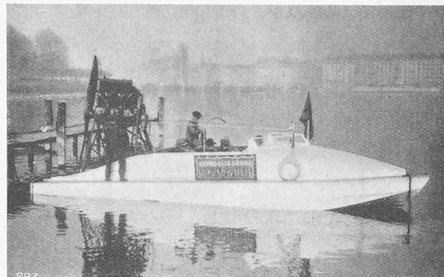
Abb. 1. Gleitboot der „S. A. des Hydro-Glisseurs Dumond-Galvin“, Paris. Tragkraft 15 Personen; 80 PS, v = 40 km/h.
