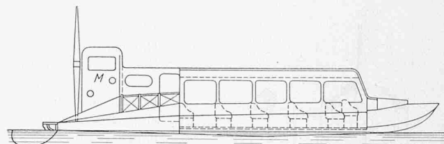
Abb. 2. 150 PS - Hydro-Glisseur; Typenskizze 1: 150. Eigengewicht 2 t, Nutzlast 2 t (20 Personen), v bis 50 km/h. Länge 12,5 m, Breite 4,0 m, Tiefgang in Ruhe 18 cm, in Fahrt 6 cm.
